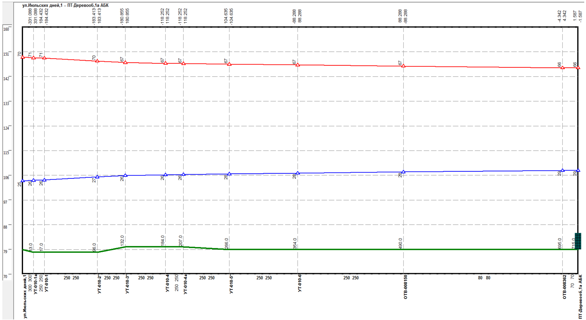
Рисунок 1.32 –Результат гидравлического расчета - график гидравлических режимов по пути теплоносителя от Июльских дней, 1 до ПТ-Деревооб, 1а АБК
