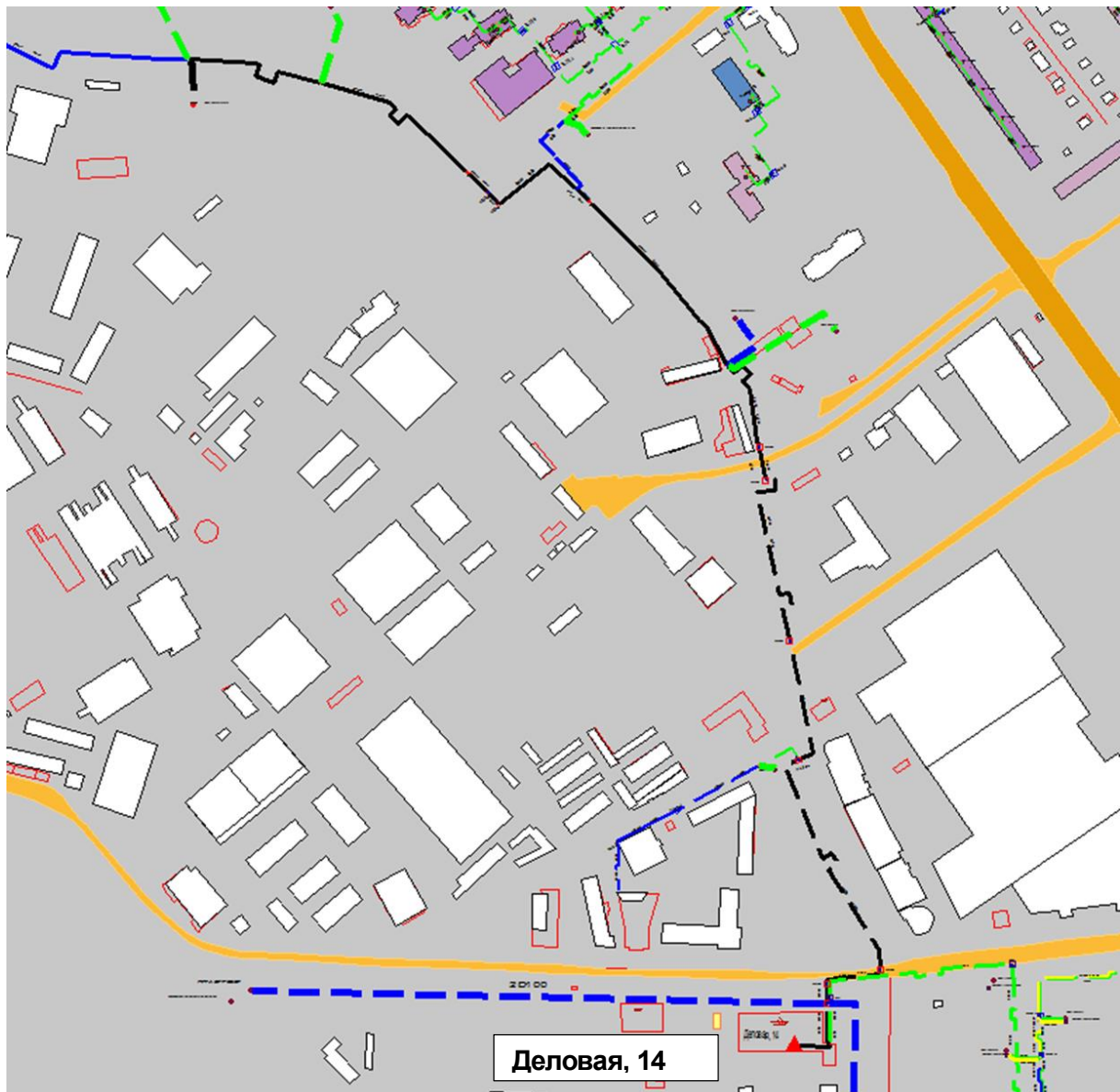
Рисунок 1.27 – Результат гидравлического расчета - расчетный путь теплоносителя от котельной Деловая, 14 до ПТ-ПП-2.99-2017-2018
