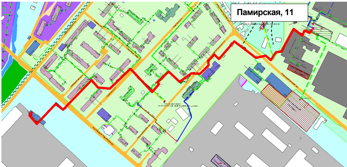
Рисунок 1.15 – Результат гидравлического расчета - расчетный путь теплоносителя от котельной Памирская, 11 до ПТ-Нахимова,3
