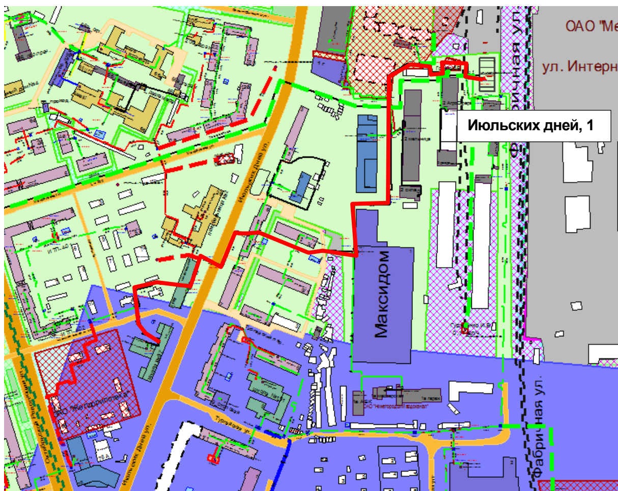
Рисунок 2.19 – Результат гидравлического расчета - расчетный путь теплоносителя от Июльских дней, 1 до ПТ-Июл.дней, 10 школа
