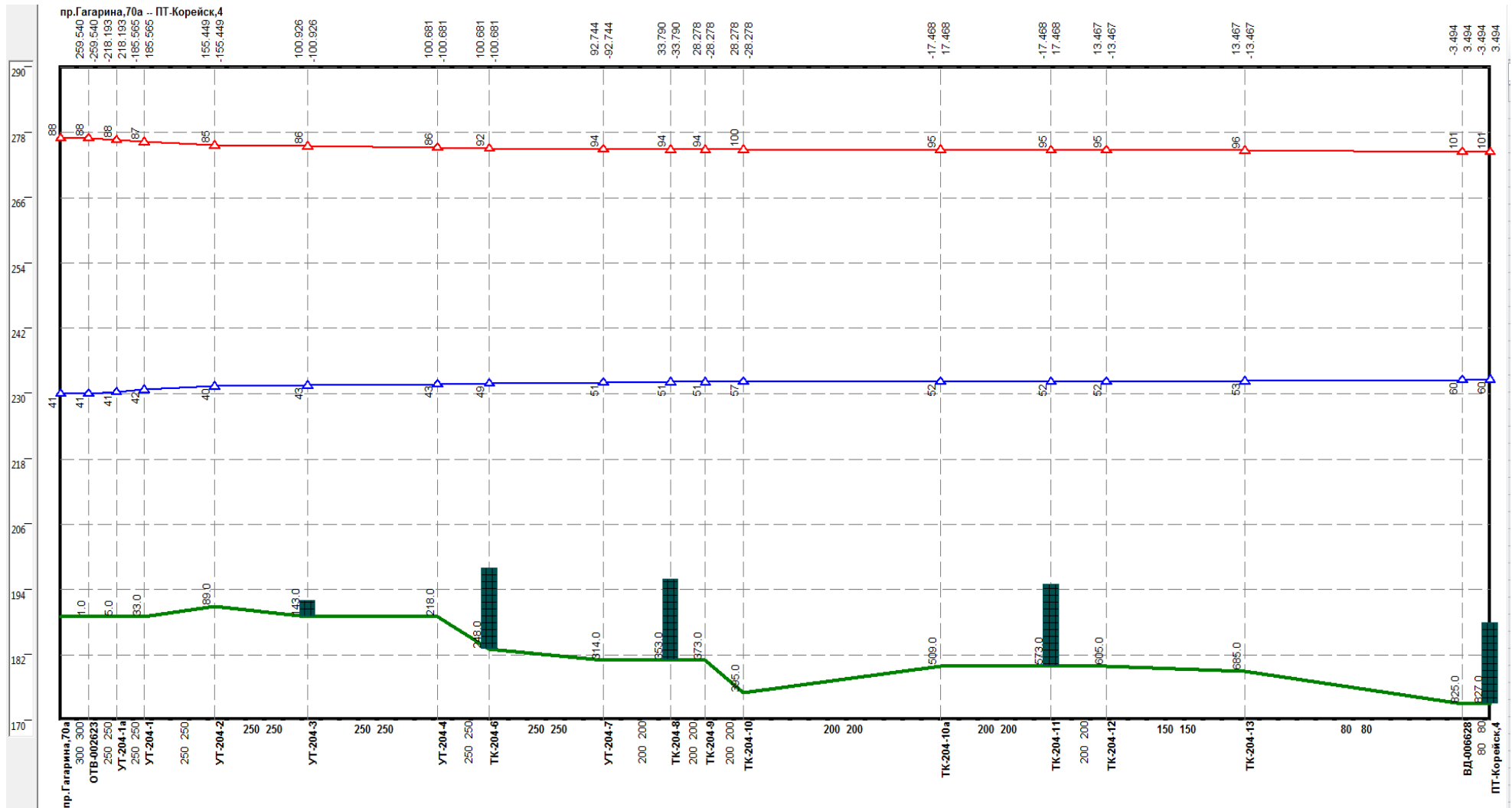
Рисунок 1.52 –Результат гидравлического расчета - график гидравлических режимов по пути теплоносителя от котельной пр. Гагарина, 70а до ПТ-Корейск,4
