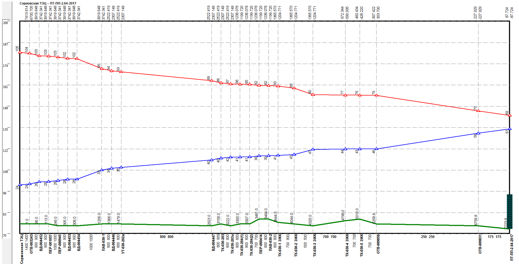
Рисунок 2.4 –Результат гидравлического расчета - график гидравлических режимов по пути теплоносителя от СтЭЦ до ПТ-ПП-2.64-2017
