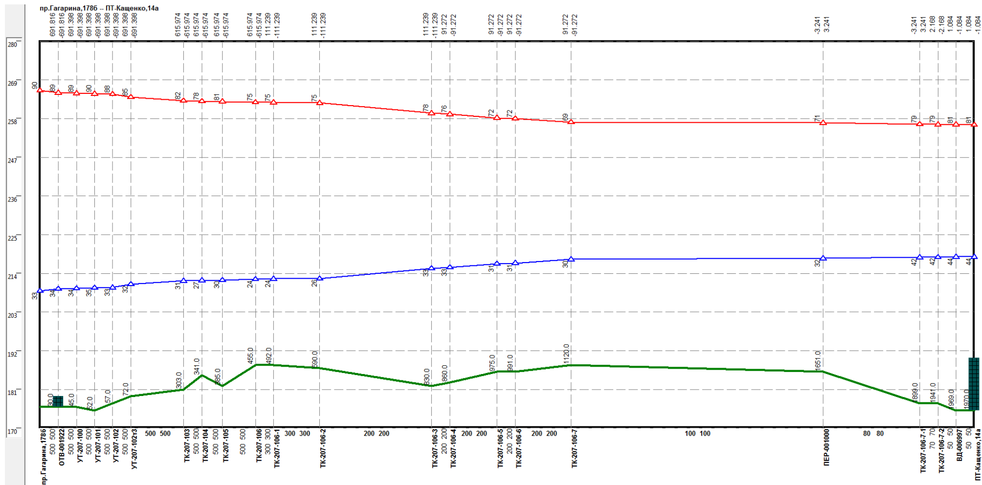
Рисунок 1.62 –Результат гидравлического расчета - график гидравлических режимов по пути теплоносителя от котельной пр. Гагарина, 1786 до ПТ-Кашенко,14а
